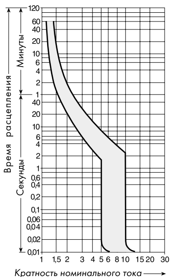
Тип мгновенного расцепления С
