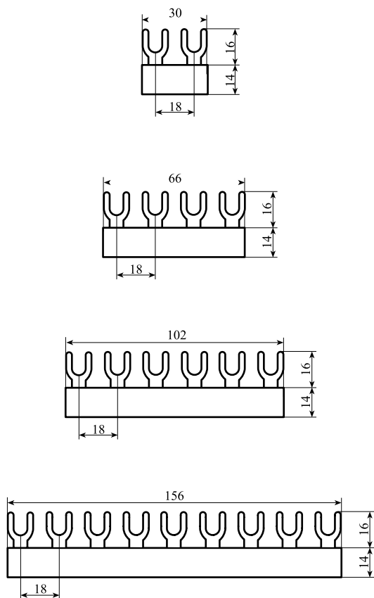
Рис. 2.8 Соединительные шины для автоматических выключателей серий 5SX2, 5SX4 и 5SX5
