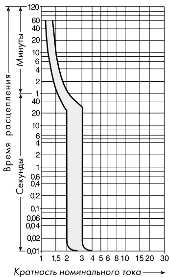
Тип мгновенного расцепления А
