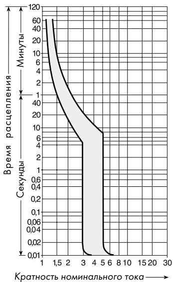
Тип мгновенного расцепления В
