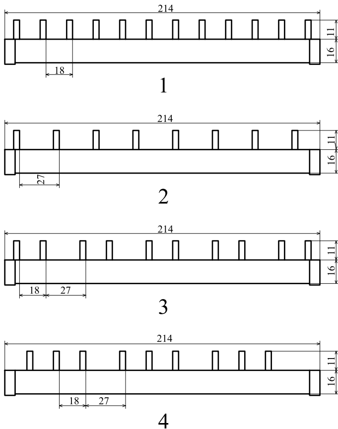
Рис. 2.13 Соединительные шины длиной 214 мм для автоматических выключателей серий 5SY4 и 5SY7 1 — одно-, двух-, трех- и четырехполюсные соответственно для одно-, двух-, трех- и четырехполюсных автоматических выключателей без БКП или БКС; 2 — однополюсные для однополюсных автоматических выключателей с БКП или БКС и трехполюсные для однополюсных автоматических выключателей с БКП или БКС; 3 — двухполюсные для двухполюсных автоматических выключателей с БКП или БКС
