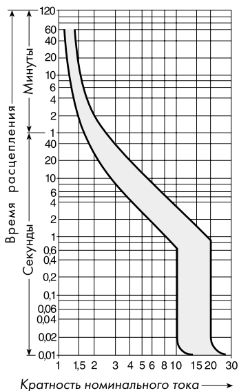
Тип мгновенного расцепления D
